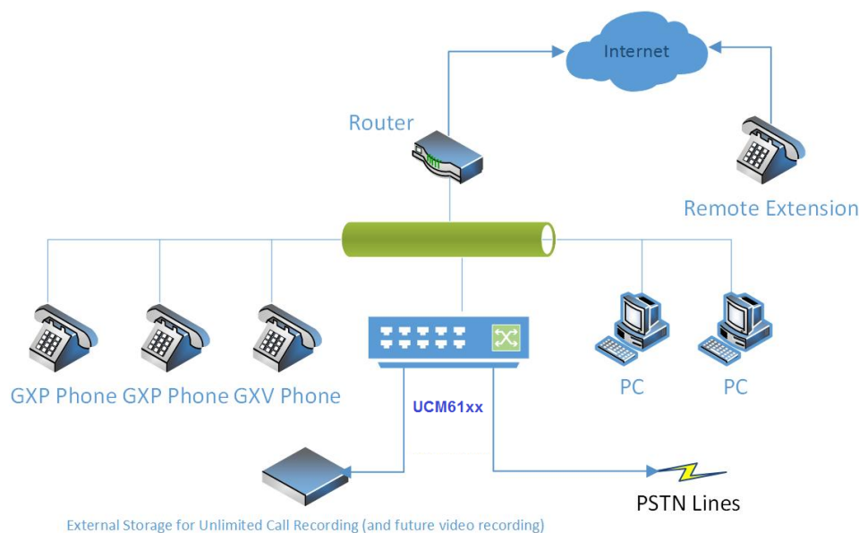
图 23 61xx 和话机在相同网络内
