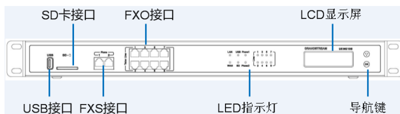
图 5: UCM6108 正面图
