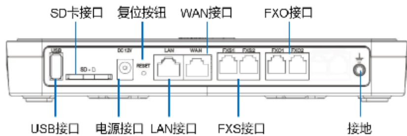
图 1: UCM6102 正面图
