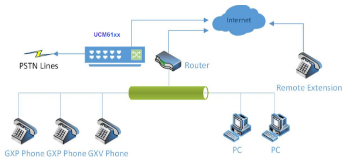
图 24 xx 和话机在不同的 LAN 网络
