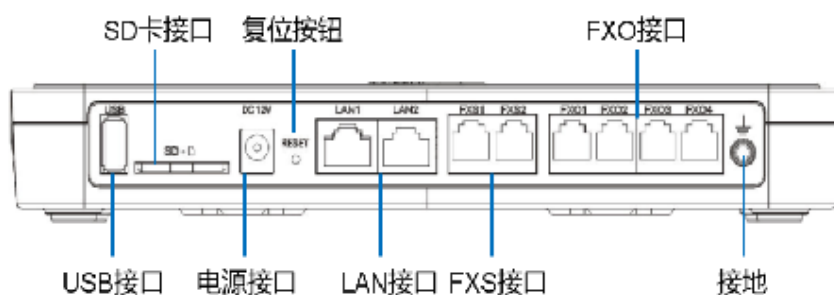
图 3: UCM6104 正面图
